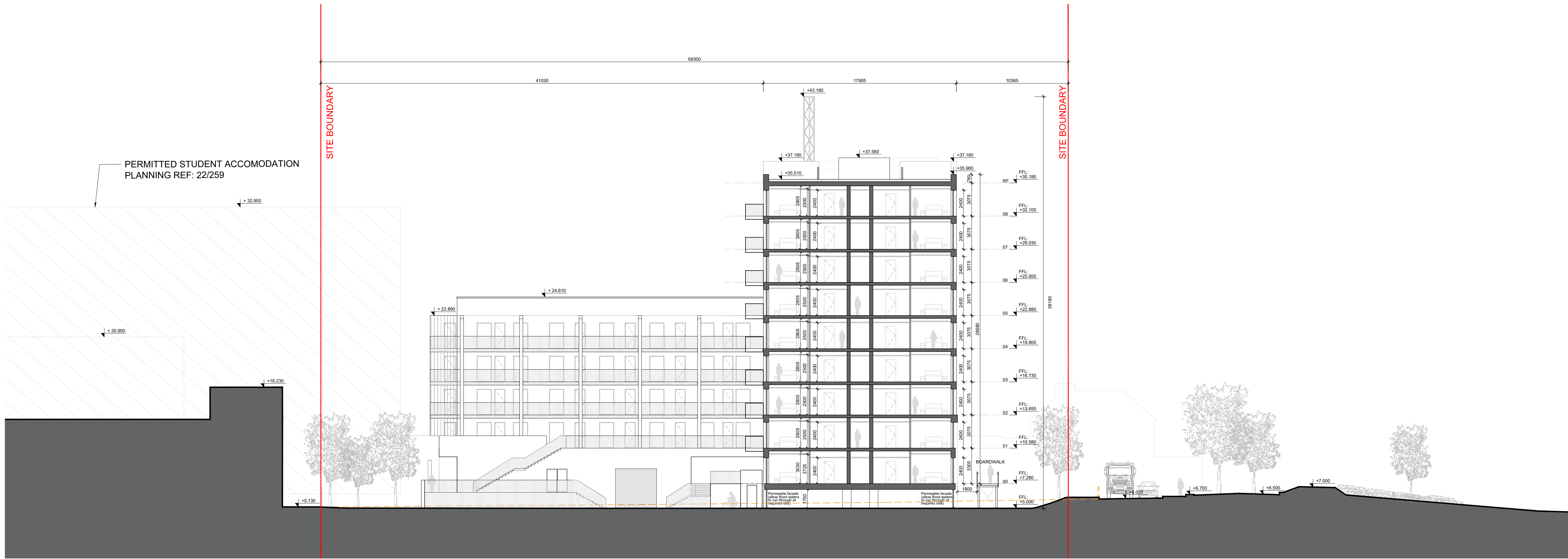
02 SECTION BB 0300 1:200 @A1
