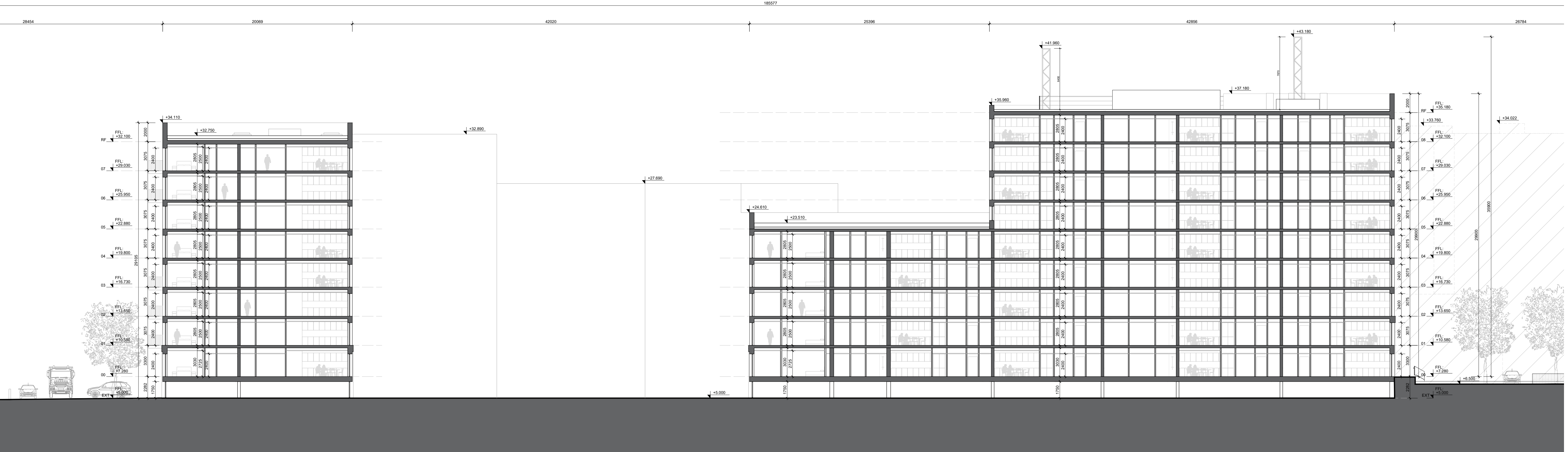
01 SECTION AA 0300 1:200 @A1
